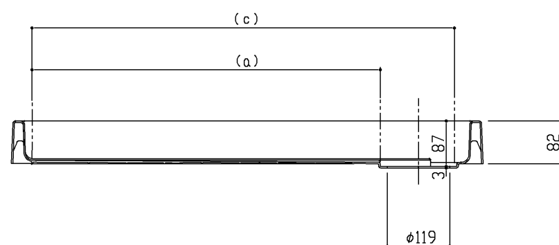
断面A-A
